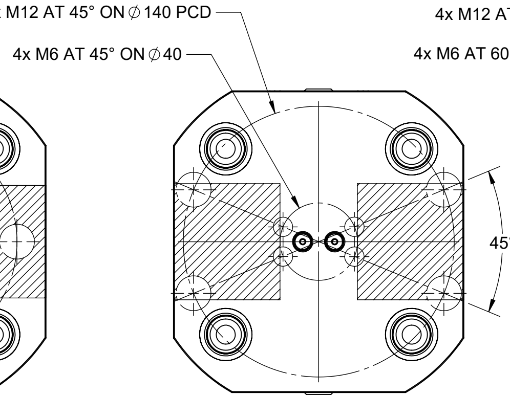
45° PATTERN
